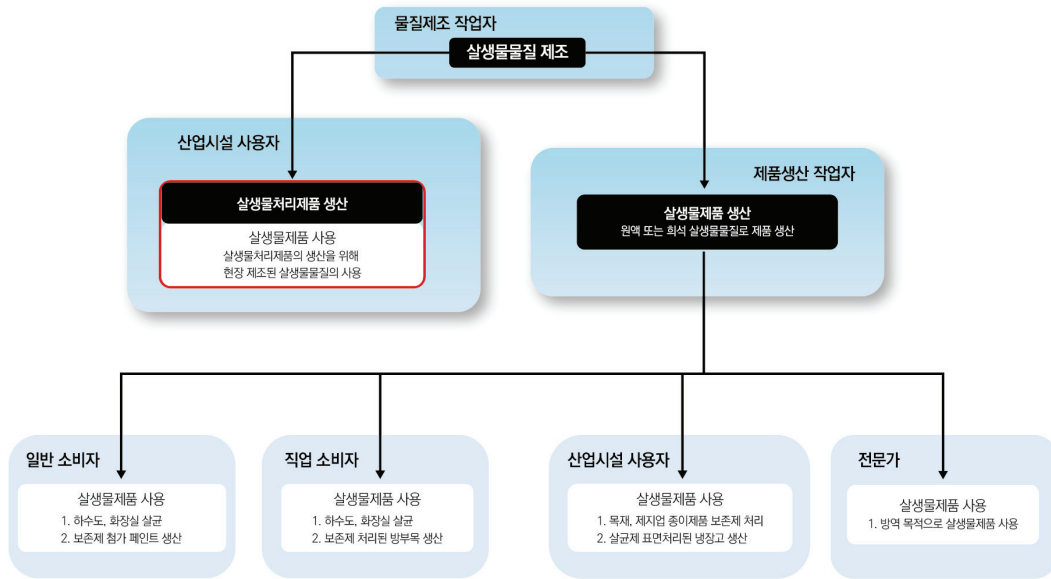
그림 5 • 살생물물질 사용주기단계
